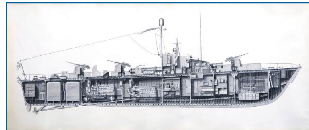
Чертежи большого торпедного катера проекта 183 У: «Продольный разрез», «План палубы и надстройки» 1950-е гг.
